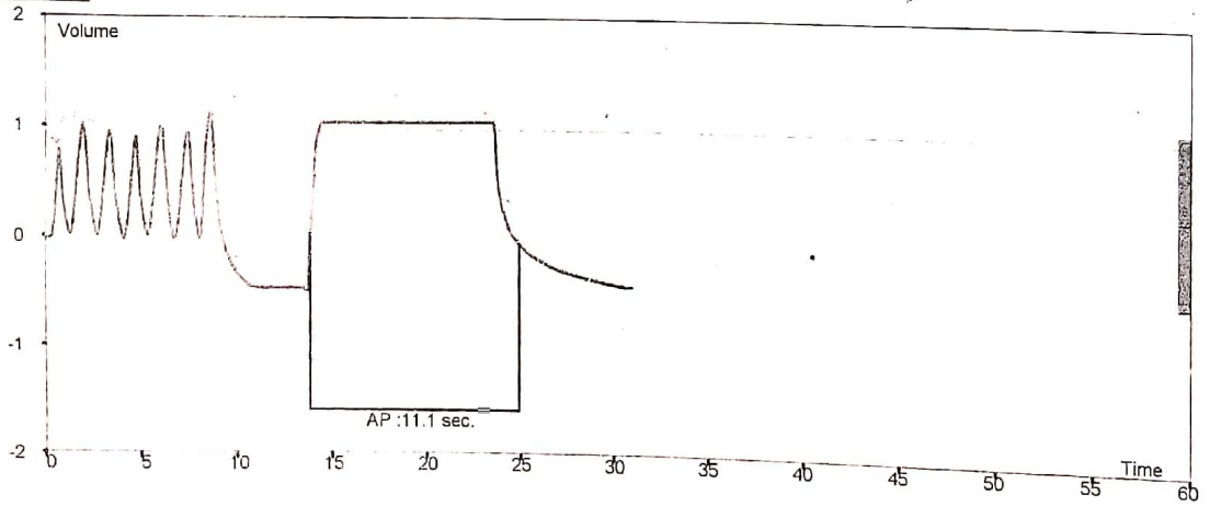
Diffusion
